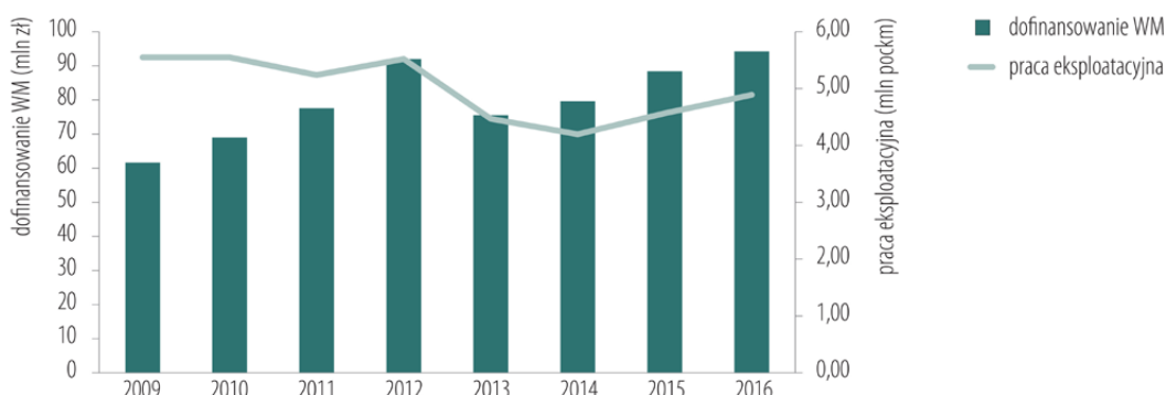
Wykres 142. Praca eksploatacyjna pociągów [w mln pociągokilometrów] oraz dofinansowanie przewozów kolejowych z budżetu województwa małopolskiego na terenie województwa małopolskiego
