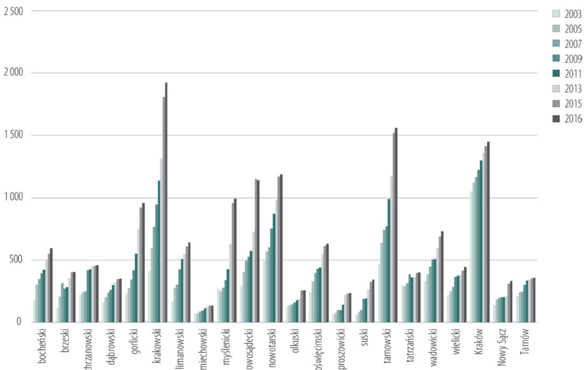
Wykres 151. Długość sieci kanalizacyjnej w województwie małopolskim (w km)
