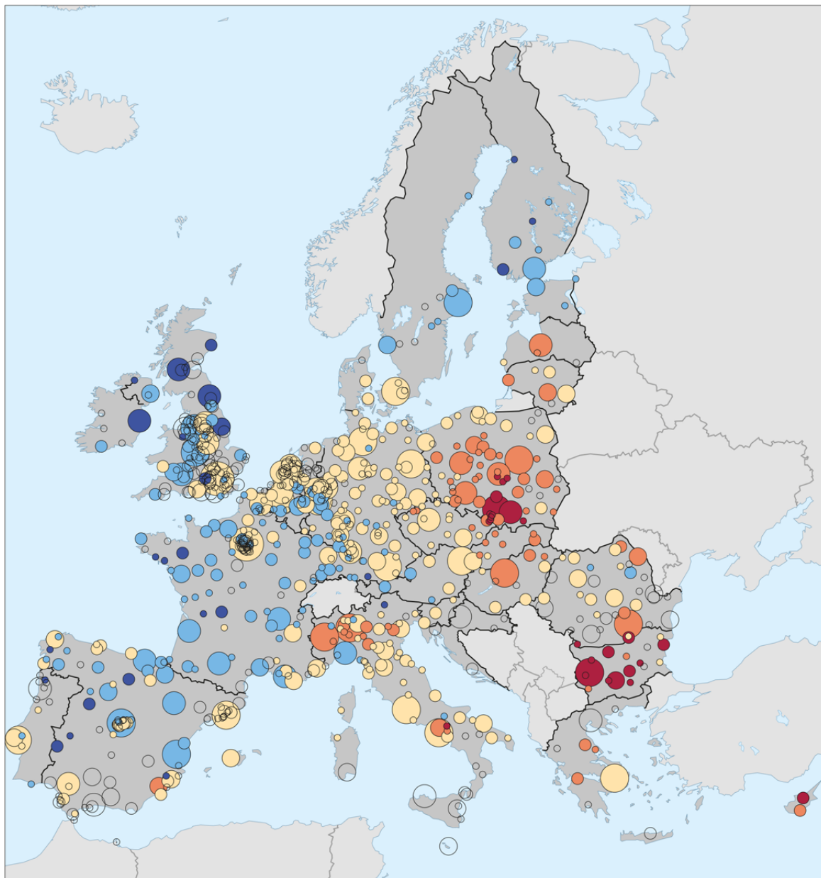
Mapa XVIII. Stężenie pyłu zawieszonego PM10 w miastach w 2014 roku
