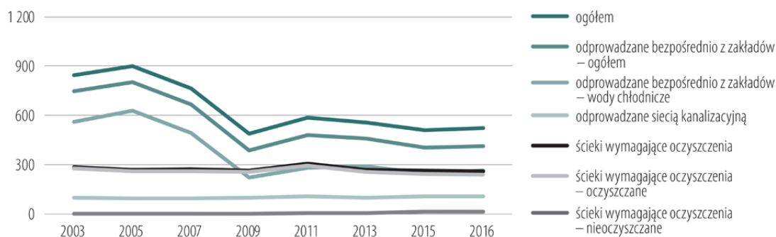
Wykres 2. Ścieki przemysłowe i komunalne odprowadzone do wód powierzchniowych lub ziemi w województwie małopolskim (hm 3 /rok)
